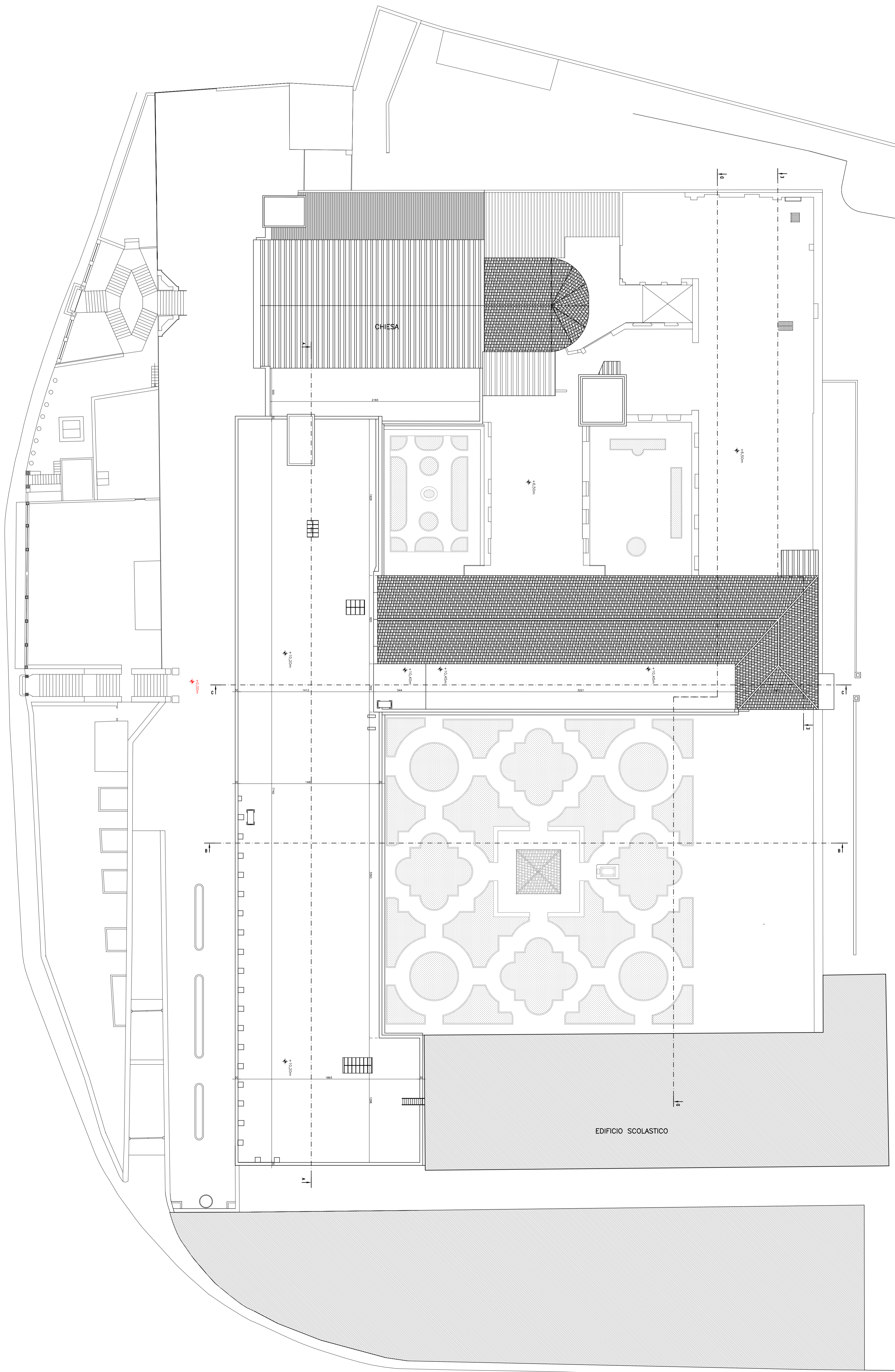
PIANTA COPERTURA Scala 1:200
