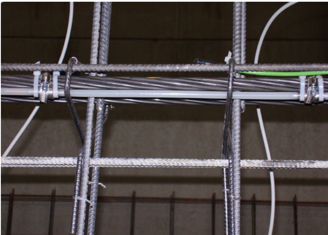
INSTALLAZIONE DEI SENSORI E DELLE TERMOCOPPIE
